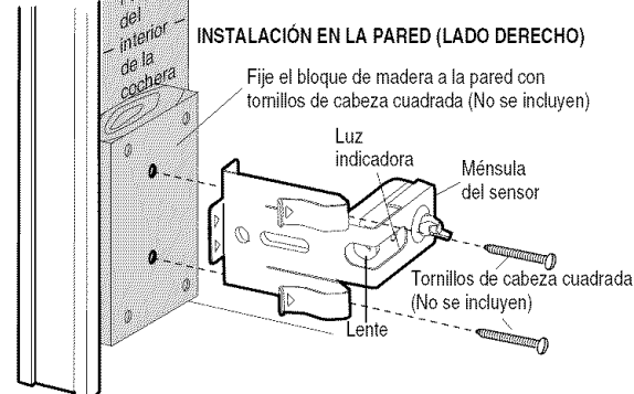
Figura 3 INSTALACIÓN EN LA PARED (LADO DERECHO)
