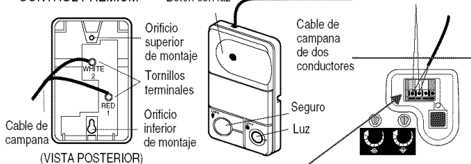
Conexiones del control de la puerta
