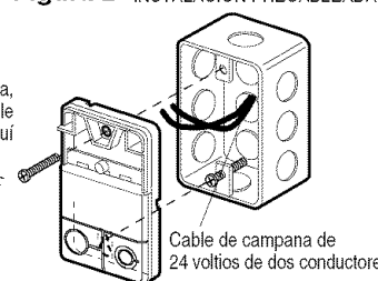
Figura 2 INSTALACIÓN PRECABLEADA
