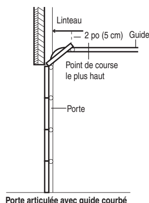
Porte articulée avec guide courbé
